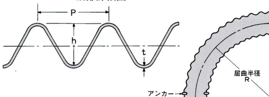
波部詳細図
